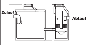
3P Hydrosystem 1000 Sternanordnung mit Voredimentation
