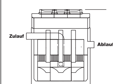
3P Hydrosystem-Drilling in Schachtbauwerk D=2,50m
